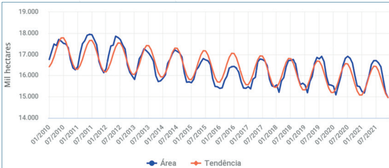
Figura 7: Série temporal mensal de superfície de água no Brasil.
