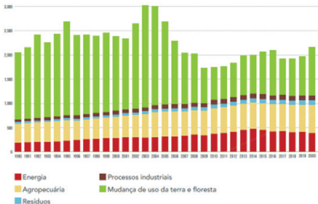
Figura 11: Emissões de gases de efeito estufa do Brasil de 1990 a 2020 (GtCO 2 e).
